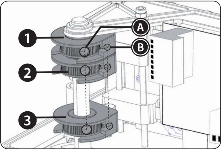
FIG. 4 MECHANICAL LIMIT SWITCH / FINECORSO MECCANICO FINS DE COURSES MECANQUES / FINAL DE CARRERA MECÁNICO MECHANISCHER ENDSCHALTER
