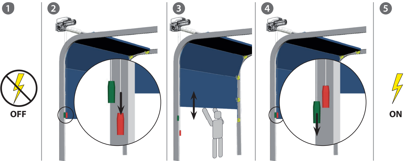
FIG. 5 MANUAL DECLUTCH / SBLOCCO MANUALE DEBRAYAGE RAPIDE / DESBLOQUEO MANUAL MANUELLE ENTRIEGELUNG / GEBRUIK VAN DE ONTKOPPELING
